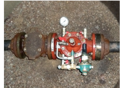
Vanne de régulation de pression (source : OIEau)
