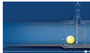
Introduction d'un hydrophone libre Smart Ball® (source : Pure Technologies)
