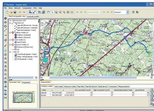
Exemple de modélisation avec le logiciel Porteau (source : Irstea)
