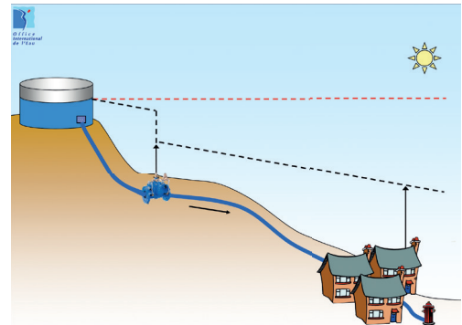
Principe de la réduction de pression (source : OIEau)
