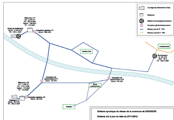
Exemple de synoptique de réseau (source : ASTEE)
