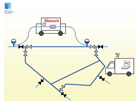
Prélocalisation par quantification par alimentation directe d'une zone (source : OIEau)
